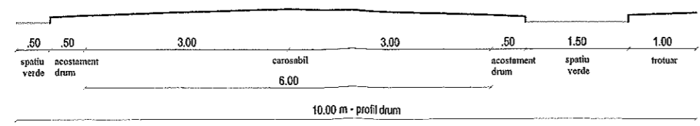
PROFIL STRADAL I-1 NOU PROPUȘ SCARA 1:50
